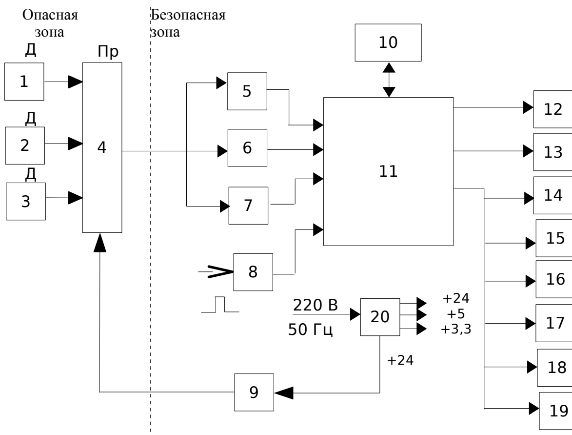
Структурная схема устройства ИП-120.
