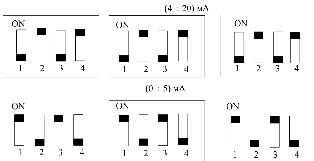
Положение DIP-переключателей
